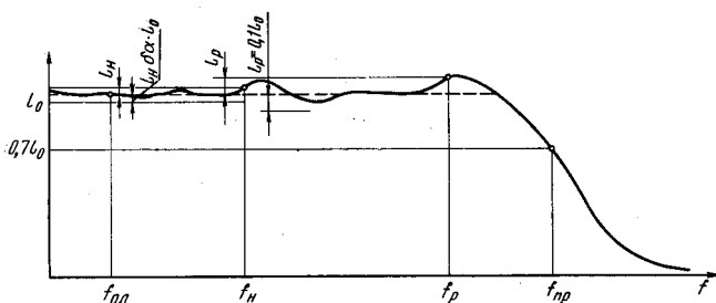
f_{оп} — опорная частота; f_n — нормальный диапазон; f_p — расширенный диапазон; f_{пр} — верхняя граница полосы пропускания; l_0 — значение АЧХ на опорной частоте; l_n — абсолютное значение неравномерности в нормальном диапазоне; l_p — абсолютное значение неравномерности в расширенном диапазоне; \delta_n — относительная погрешность коэффициента отклонения
