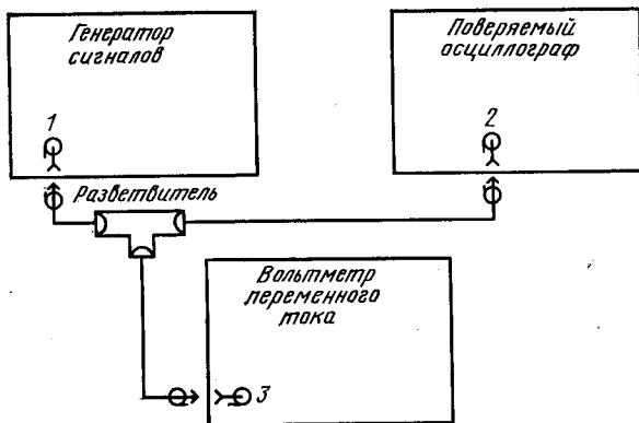
1—выход генератора сигналов; 2—вход усилителя U ; 3—вход вольтметра переменного тока
