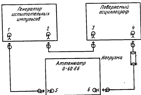
1—выход основных импульсов; 2—выход синхронизирующих импульсов; 3—вход синхронизации; 4—вход усилителя U ; 5—вход аттенюатора; 6—выход аттенюатора
