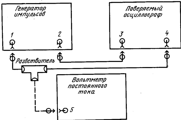
1—выход основных импульсов; 2—выход синхронизирующих импульсов; 3—вход синхронизации; 4—вход усилителя \mathcal{U} ; 5—вход вольтметра
