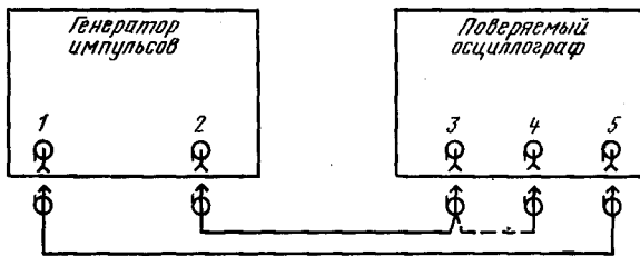
1—выход синхронизирующих импульсов; 2—выход основных импульсов; 3—вход усилителя Y ; 4—выход калибратора осциллографа; 5—вход синхронизации
