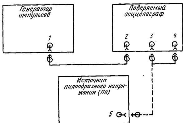
Черт. 3
