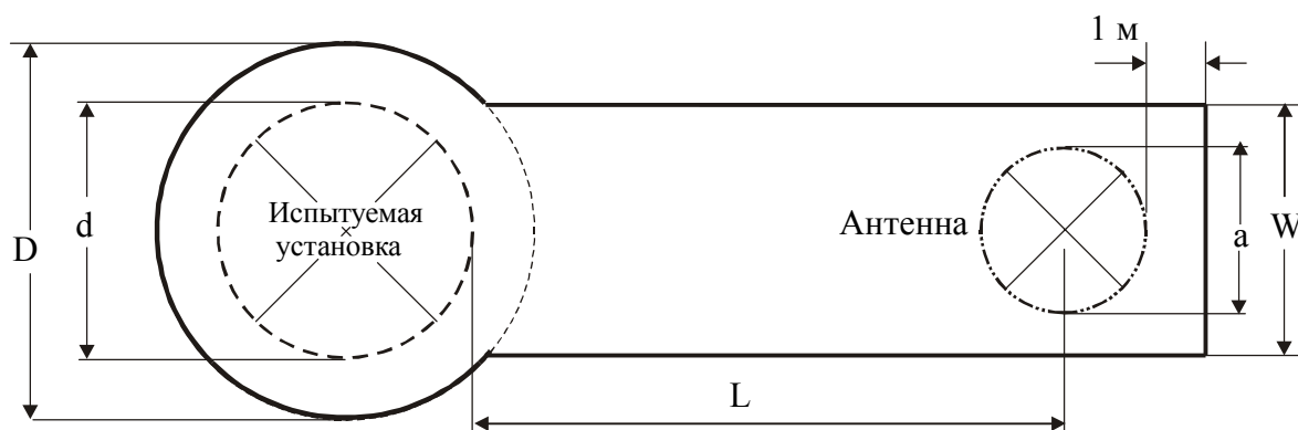
Рисунок 1 – Измерительная площадка
