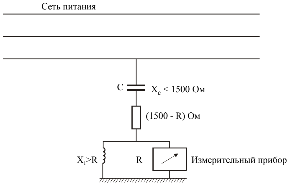
Рисунок 4 - Схема измерения напряжения ИРП на сетевых зажимах по 6.2.3
